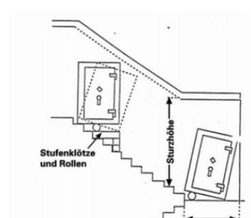
Cales et galets de marches, hauteur linteau, profondeur palier
